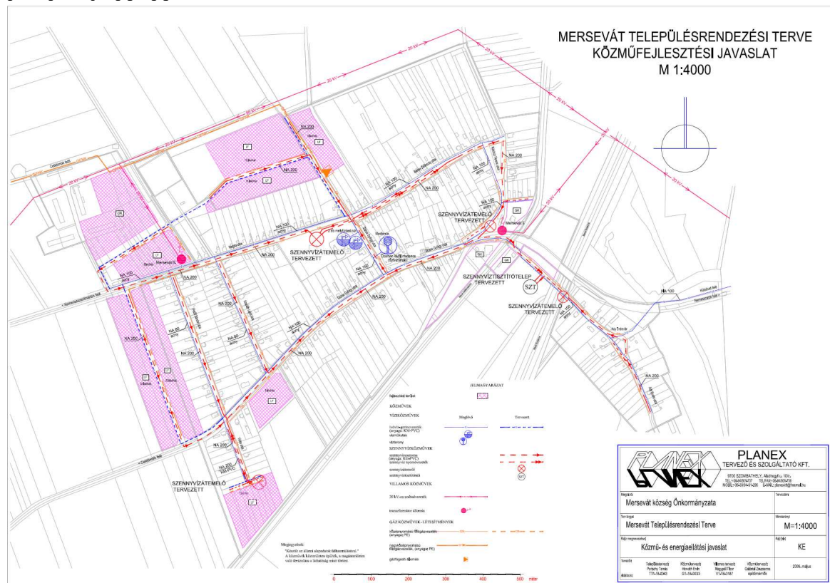
Közműellátási javaslat 2007-es rendezési tervből
