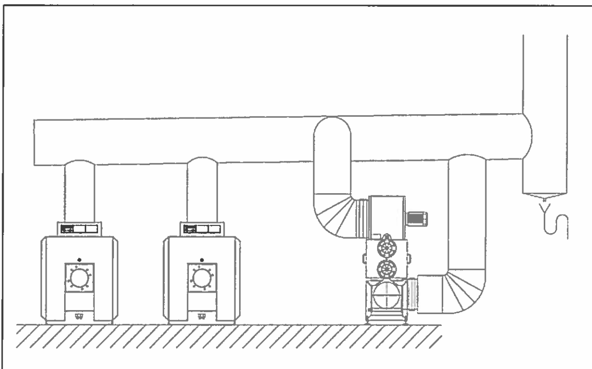
A berendezés csatlakozása a füstcsatornához
